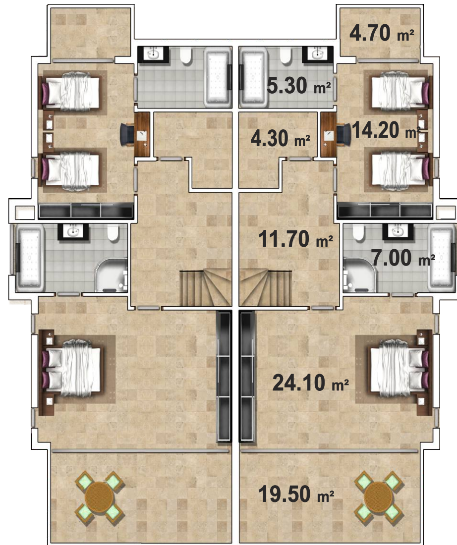
Второй Этаж
