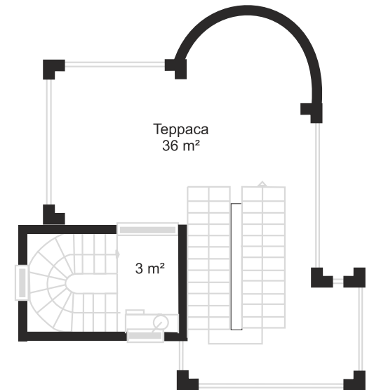
ТЕРРАСА
