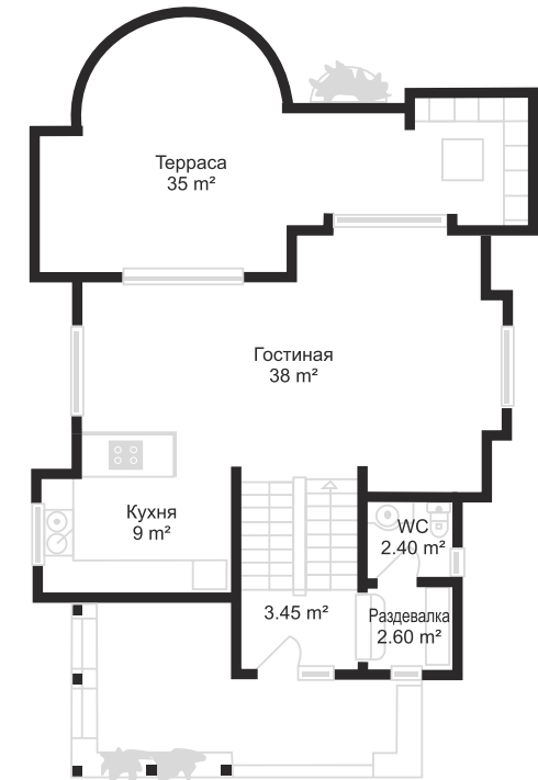
ПЕРВЫЙ ЭТАЖ
